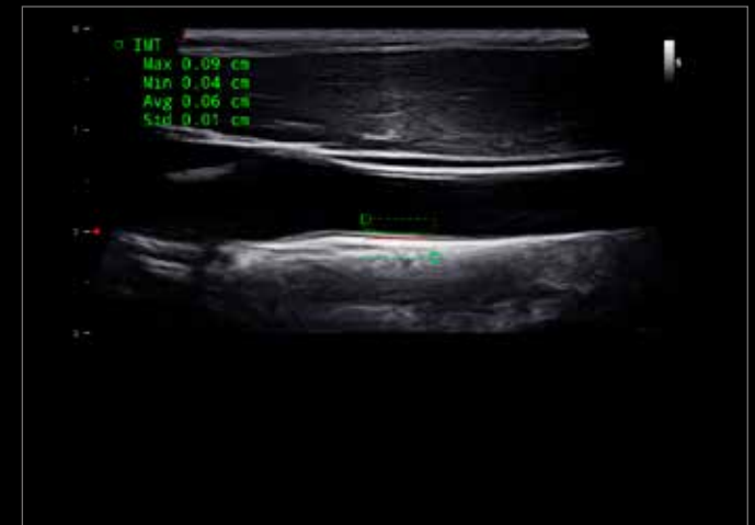
Karotis, IMT-Berechnung
